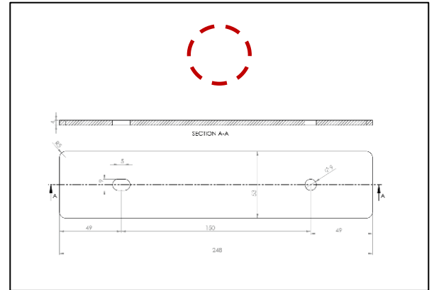
Samlebeslag varenr: 26381
